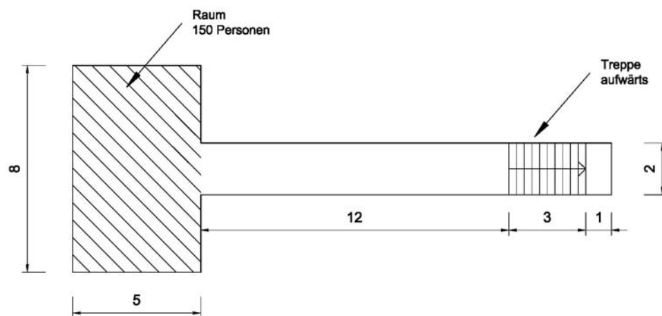
Abbildung A5: Rettungsweg über Treppe (Einheit: m)
